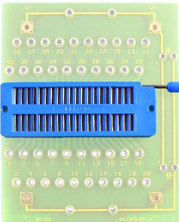
Abb. 2: Nullkraft-Spannfassung
