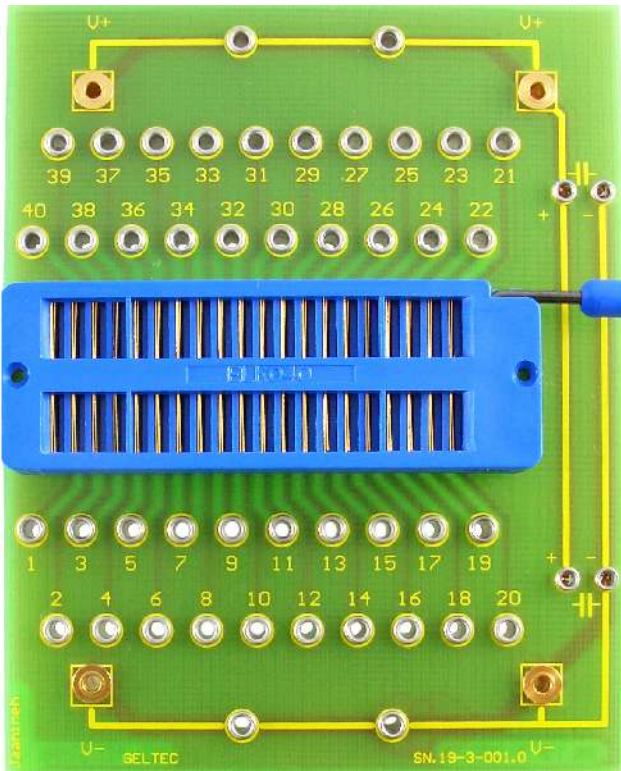
Abb. 1: Draufsicht Spannfassungskarte
