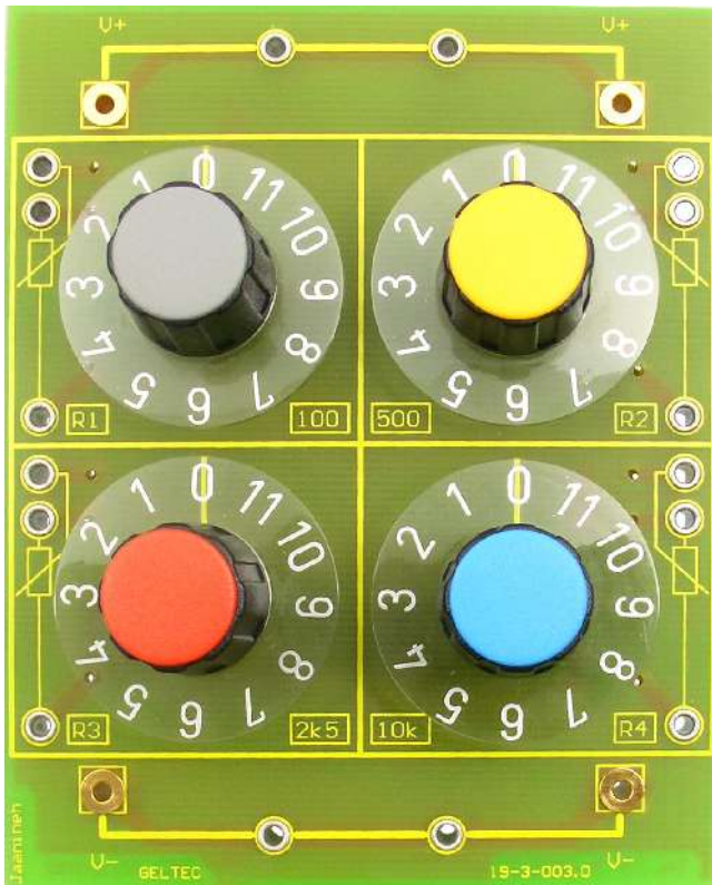
Abb. 1: Draufsicht Vierfach-Leistungspotikarte
