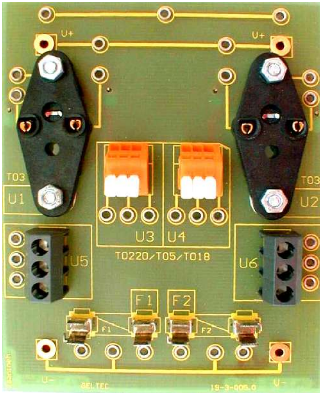
Abb. 1: Draufsicht Leistungshalbleiterkarte
