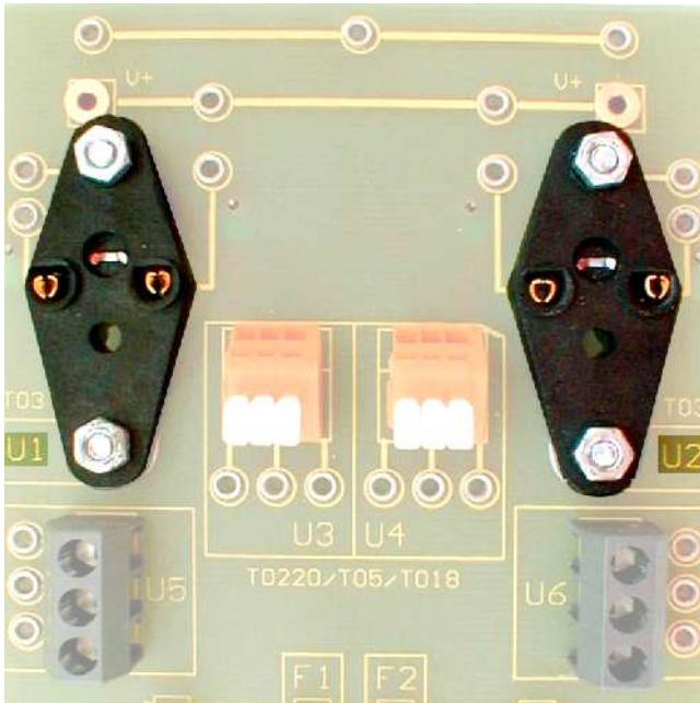
Abb. 4: Fassung U1, U2
