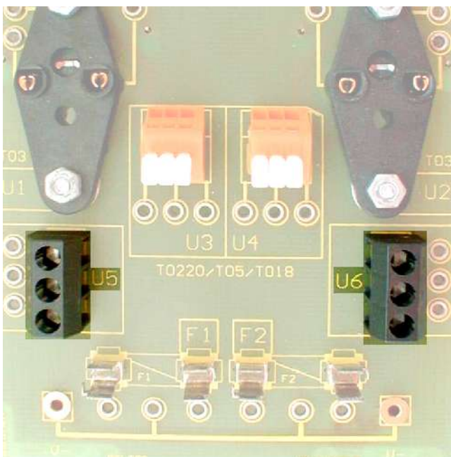
Abb. 3: Fassung U5, U6
