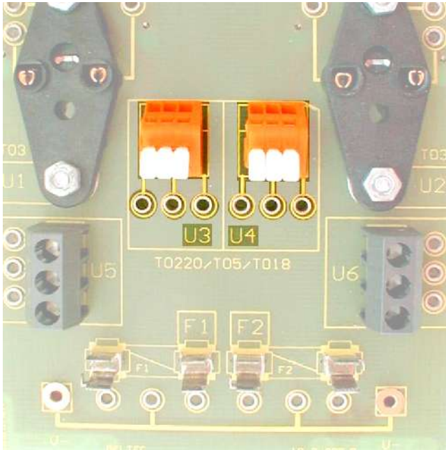
Abb. 2: Fassung U3, U4
