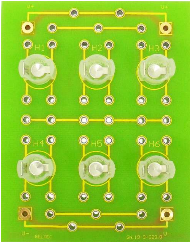
Abb. 1: Draufsicht Sechsfach-Glühlampenkarte
