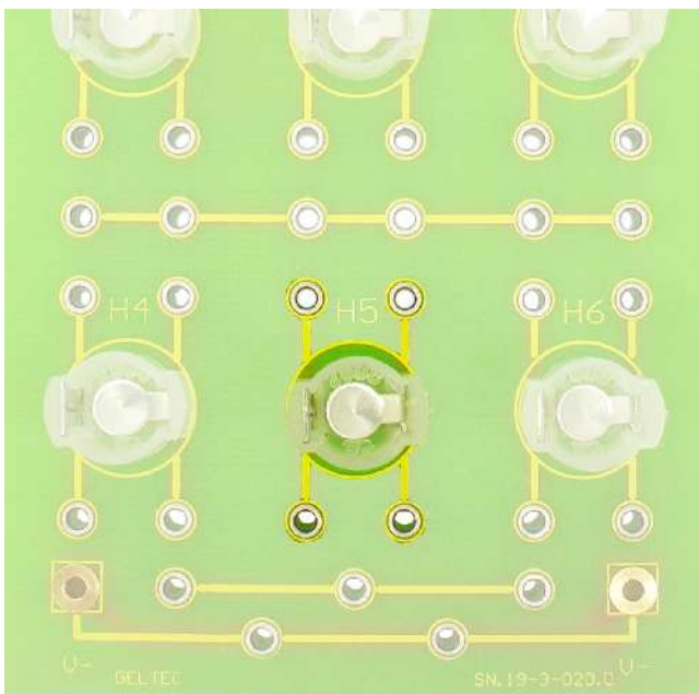
Abb. 2: Lampenfassung
