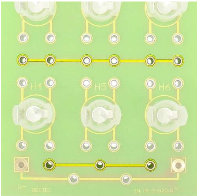
Abb. 3: Verteiler
